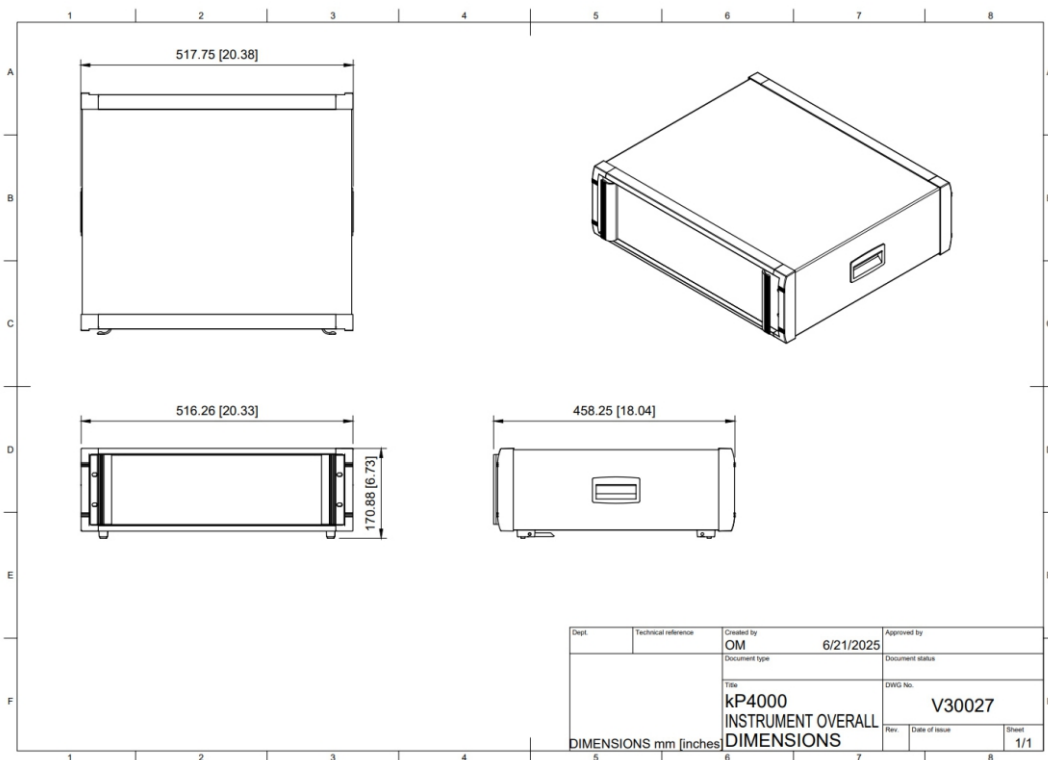
KP4226 Dimensions
